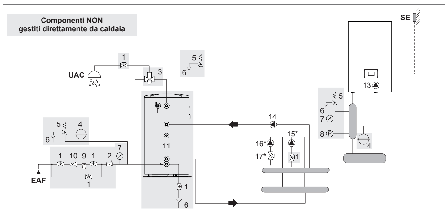
Schema 4: circuito con caldaia collegata con serbatoio A.C.S. e con impianto di riscaldamento tramite separatore
