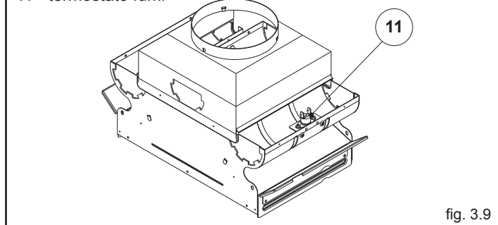
11 - termostato fumi
