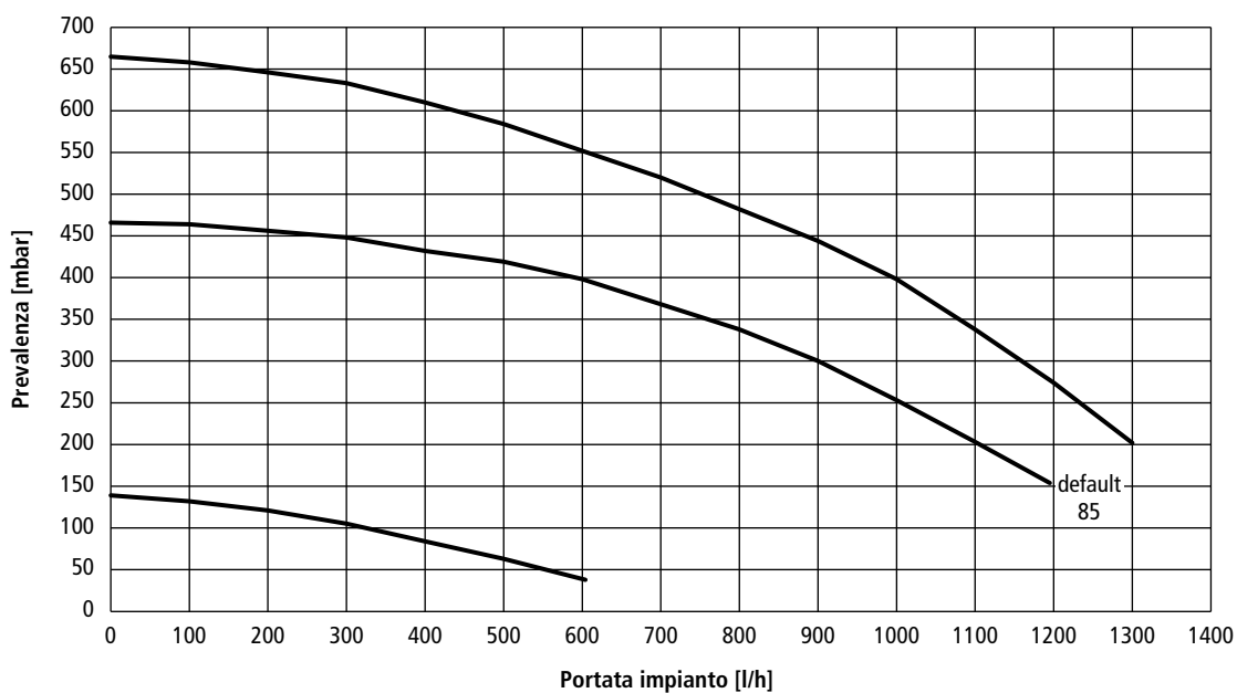
Circolatore 7 m (accessorio)
