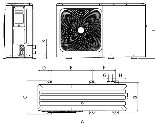
8/10/12/14/16 kW (jednostka: mm)
