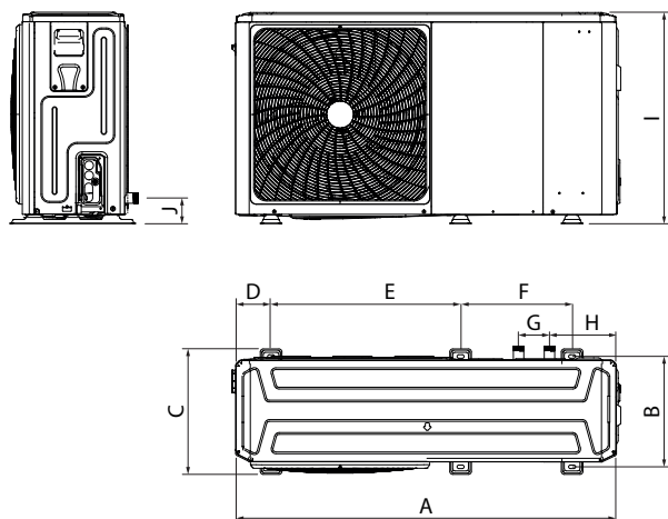
4/6 kW (jednostka: mm)
